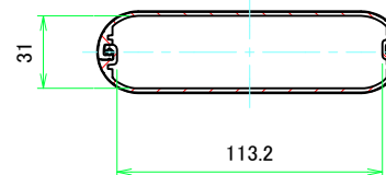
A-A (1:2.5)
